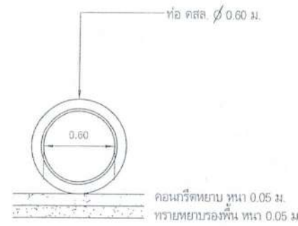
รูปตัดท่อระบายน้ำ 1 : 25
