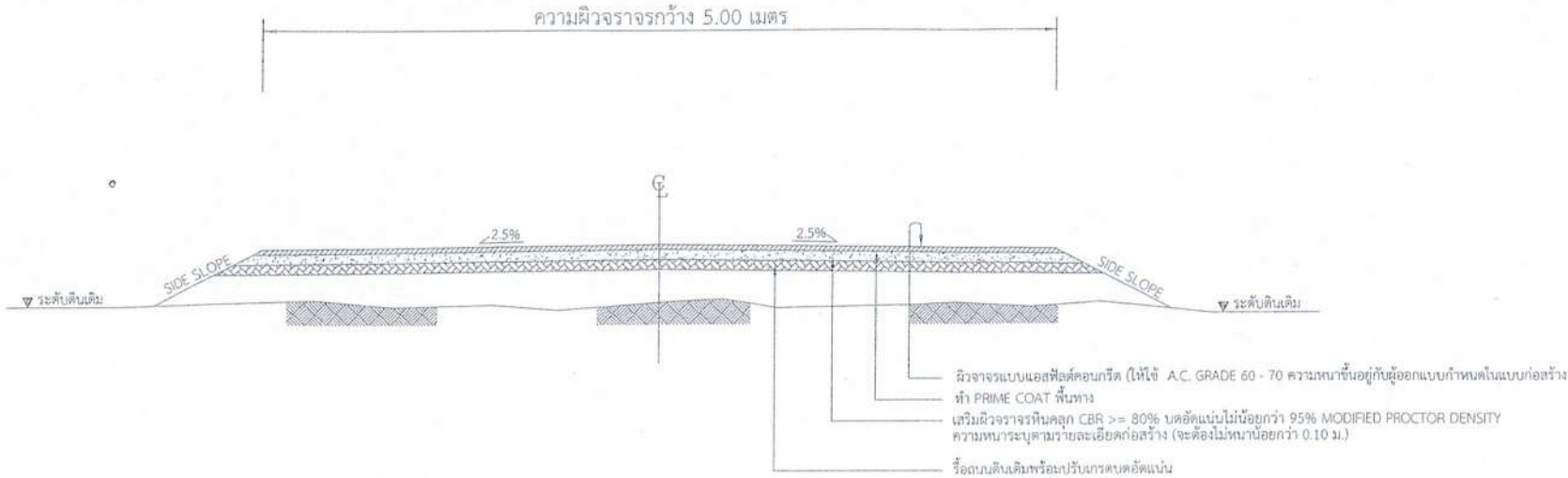
รูปตัดตามขวาง ช่วงที่ 2 กม. 1+410 ม. - กม. 2+920 ม. ขนาดกว้าง 5.00 ม. ระยะทาง 1,510.00 ม. หนา 0.05 ม.
